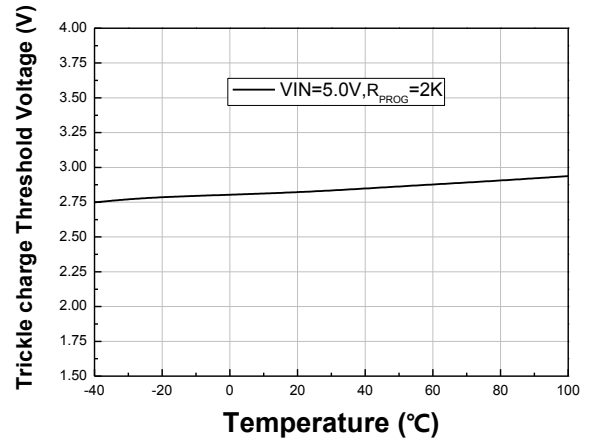
16. 涓流充电极限电压 VS 温度
