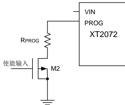
图 2. XT2072 的使能设计
